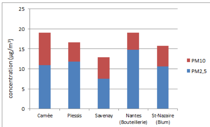
Figure 2: concentrations moyennes de PM_{10} et PM_{2,5} (courbes cumulées) dans l'environnement de l'établissement et en situation de fond urbain à Nantes et Saint-Nazaire du 15 janvier au 31 mai 2016 (excepté pour Savenay, du 15 janvier au 3 mars 2016).
