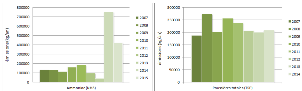
émissions atmosphériques d'ammoniac (NH3) et poussières totales (TSP) de Yara estimées de 2007 à 2015 (source : www.pollutionsindustrielles.ecologie.gouv.fr/IREP ).
