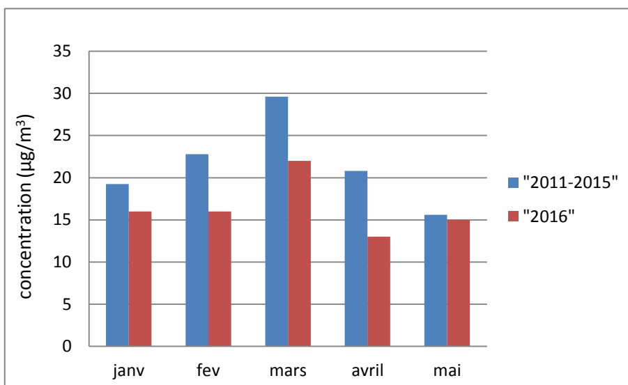
Figure 3: concentrations de PM10 en moyenne de janvier à mai ces 5 dernières années en comparaison aux concentrations de l'année 2016 à Donges (site Parscau du Plessis).
