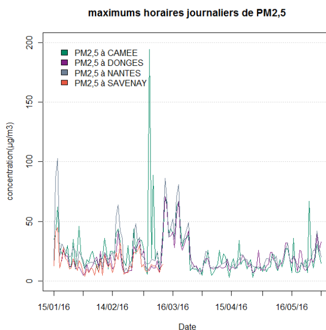
Graphique 2 : évolution des concentrations de PM 2,5 dans l'environnement de Yara, à Savenay et Nantes.
