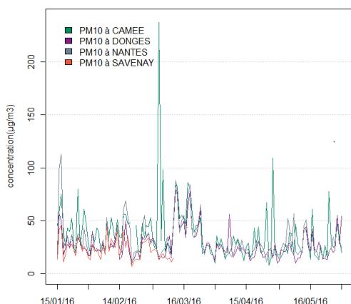
évolution des maximums horaires journaliers de PM10 dans l'environnement de Yara, à Savenay et Nantes
