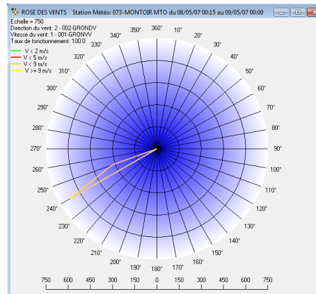
Rose de vents à Montoir de Bretagne le 8 mai 2007.
