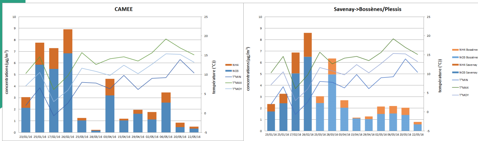
Concentrations de NO 3 et NH 4 en fonction de la température (minimale, maximale et moyenne journalière).
