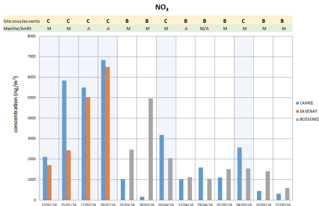
évolution des concentrations de nitrate dans l'environnement de l'établissement
