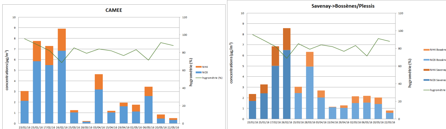
Concentrations de NO 3 et NH 4 en fonction de l'humidité relative journalière.
