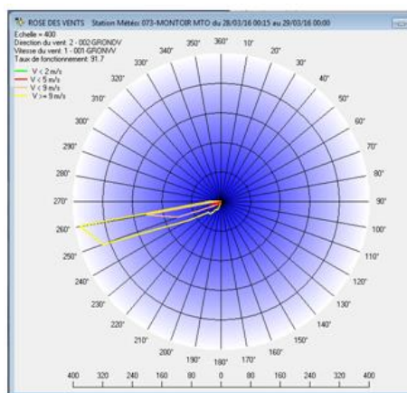
Rose de vents à Montoir de Bretagne le 28 mars 2016.
