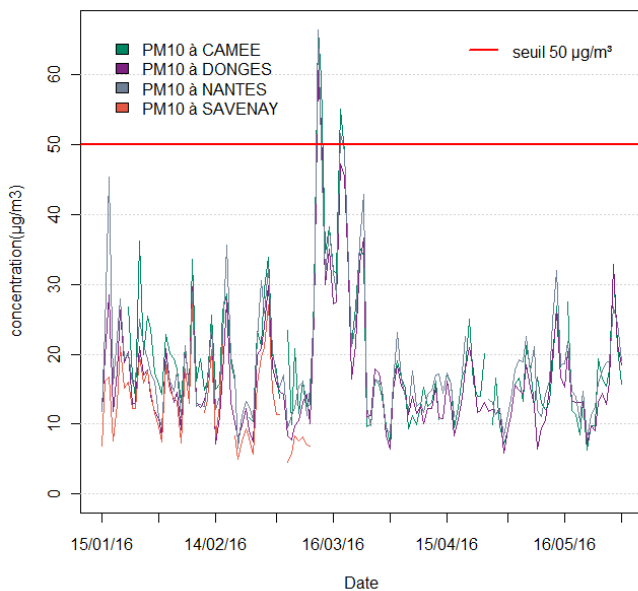
évolution des moyennes journalières de PM10
