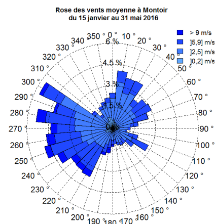
Rose des vents à Montoir durant la campagne de mesure, du 15 janvier au 31 mai 2016.
