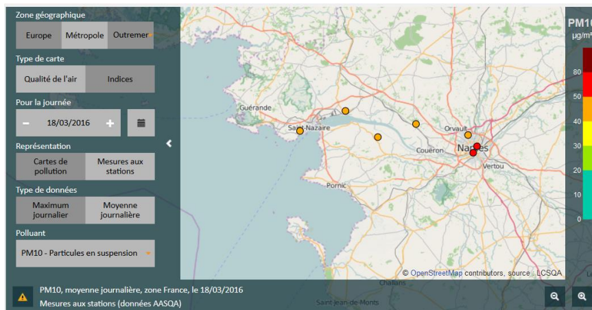
Cartes des mesures de PM10 aux stations les 12,13 et 18 mars 2016 (source : Air Pays de la Loire /Prev'air)
