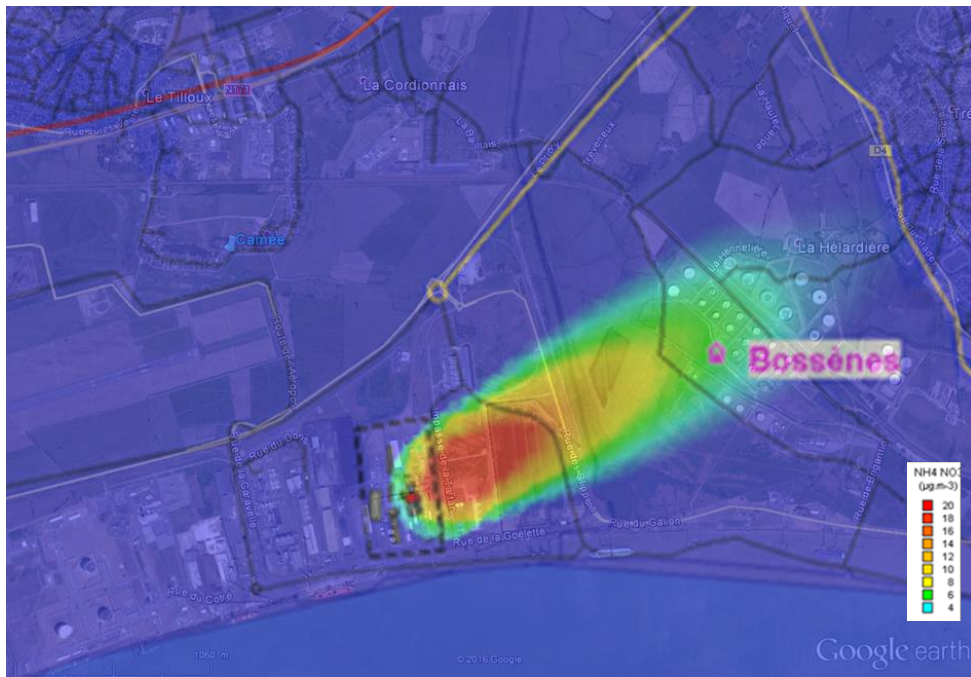
Concentrations journalières de PM1 modélisées en provenance de la tour de prilling avec le scénario d'émissions réelles de 2008 le 8 mai 2007 (vent de sud-ouest majoritaire avec une vitesse moyenne de 6,9 m.s-1)
