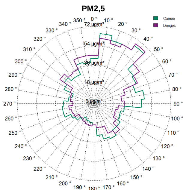
Roses de pollution des niveaux de pointe de PM2,5 (P98) du 15 janvier au 31 mai 2016.
