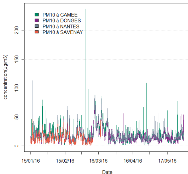
évolution des concentrations horaires de PM10
