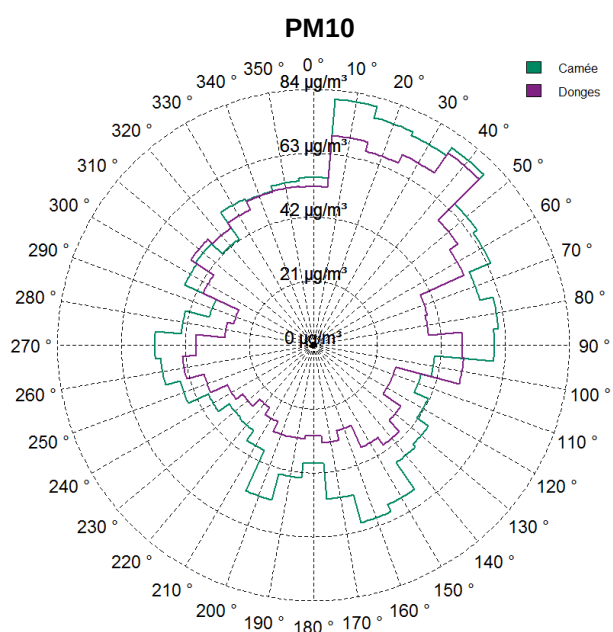
Roses de pollution des niveaux de pointe de PM10 (P98) du 15 janvier au 31 mai 2016.
