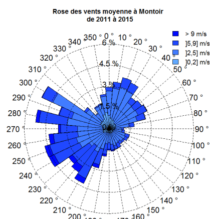
Rose des vents à Montoir en moyenne de 2011 à 2015.
