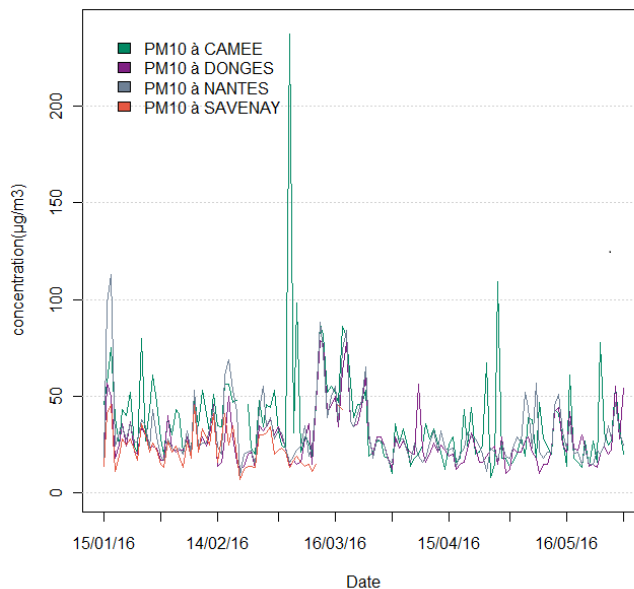
maximums horaires journaliers de PM10
