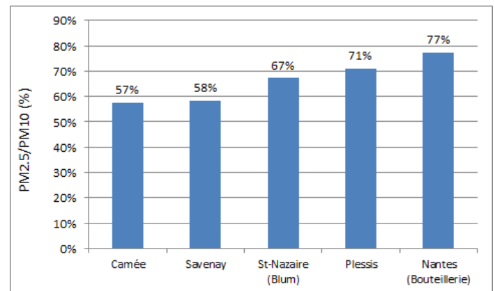
Figure 1: évolution du rapport PM_{2,5}/PM_{10} dans l'environnement de l'établissement et en situation urbain de fond du 15 janvier au 31 mai 2016 (excepté pour Savenay, du 15 janvier au 3 mars 2016).
