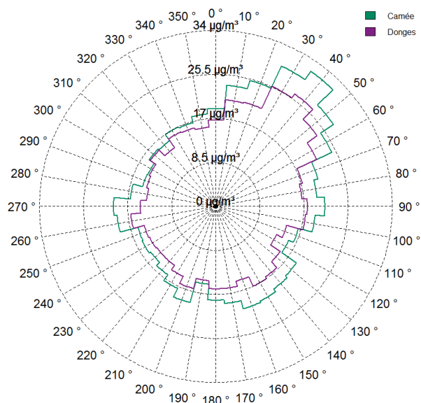
Roses de pollution moyenne PM10 du 15 janvier au 31 mai 2016.
