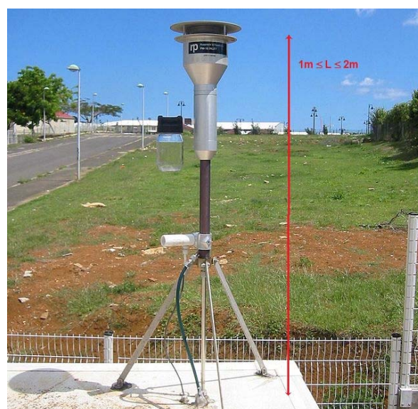
Figure 5: Exemples de configuration de point de prélèvement en toiture de bâtiment (canne de prélèvement gaz – à gauche –, tête PM – à droite)
